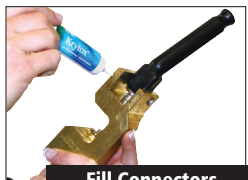
Fill Connectors
